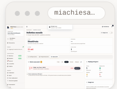
Fig. 3 Dettagli errore mostra «facebook: token scaduto». La cattura non rilancia l'automazione.
