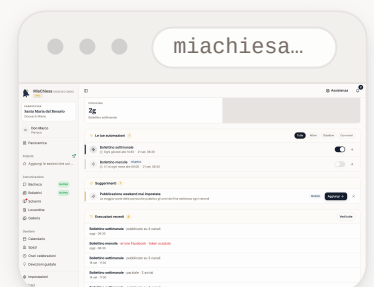
Fig. 2 Il suggerimento spiega il caso rilevato e offre Aggiungi; la cattura non ha ancora aperto la procedura.
