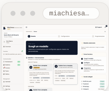
Fig. 2 In English mode, the wizard keeps the Italian heading Scegli un modello; the visible Bollettino + Avviso templates appear beside the empty summary, Come funziona and Canali collegati.
