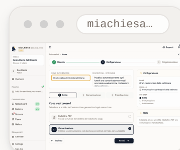
Fig. 3 The selected template opens Configurazione and pre-fills the Italian Nome automazione field.
